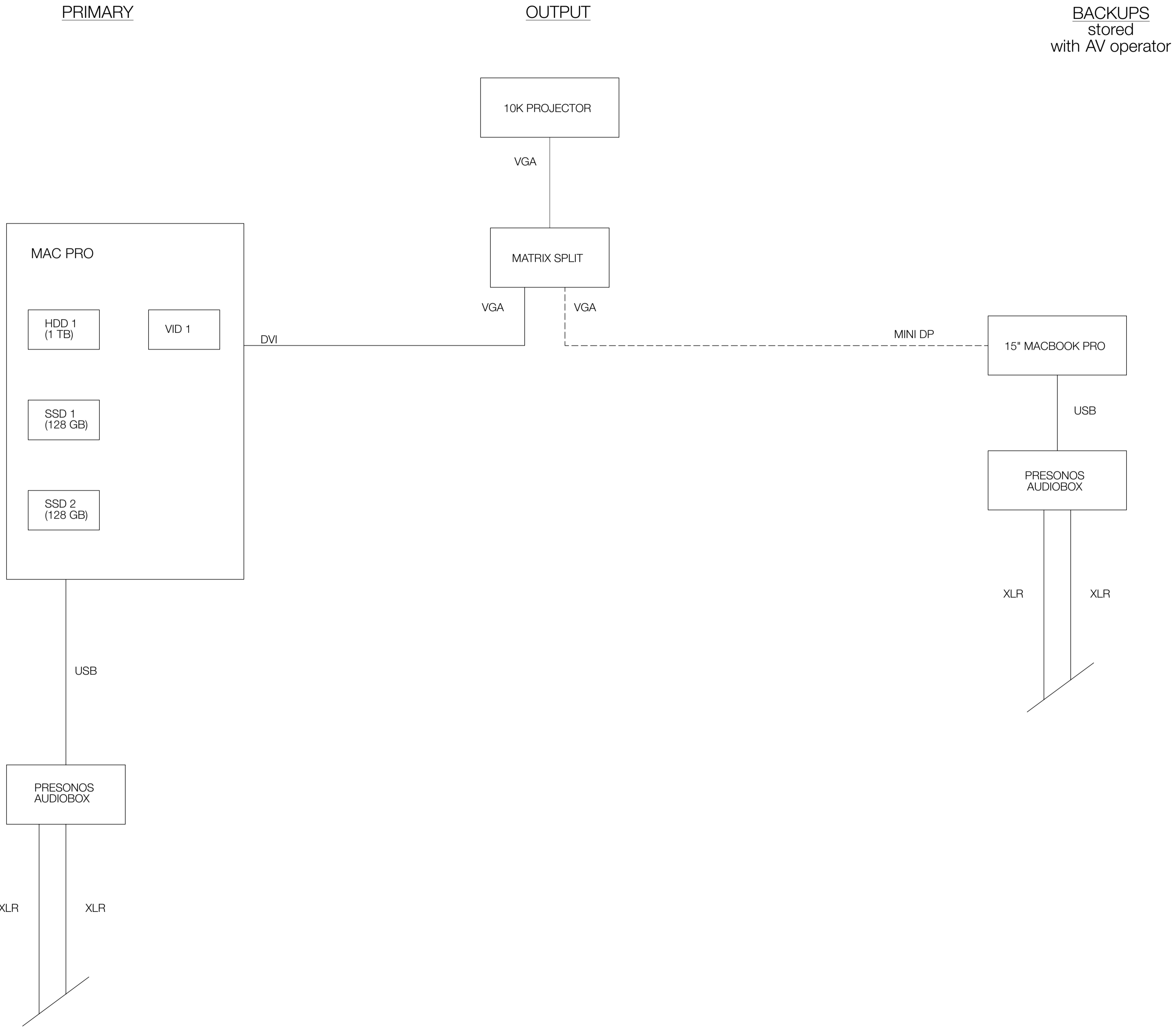
1 AV SCHEMATIC SL03-02 NOT TO SCALE
